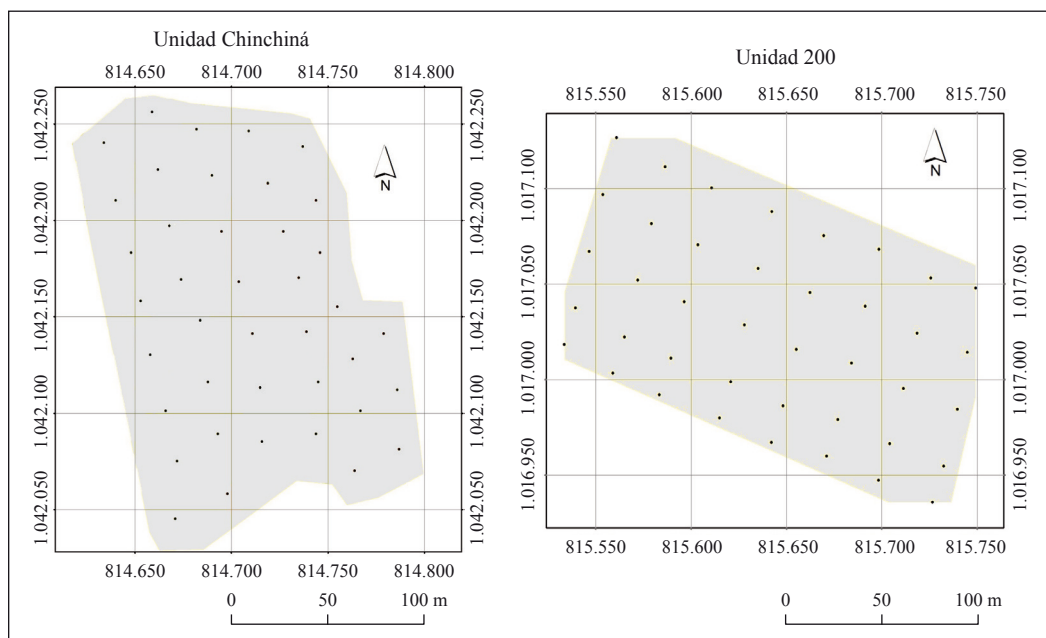
Figura 1. Distribución de los sitios de muestreo donde se midió la Da en cuatro profundidades del perfil.
