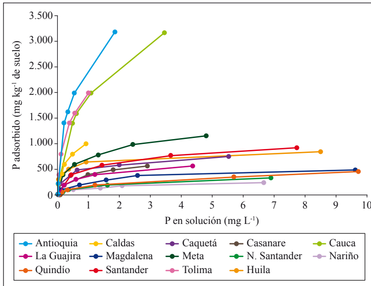
Figura 1. Isotermas de adsorción de P de suelos representativos de la zona cafetera de Colombia.
