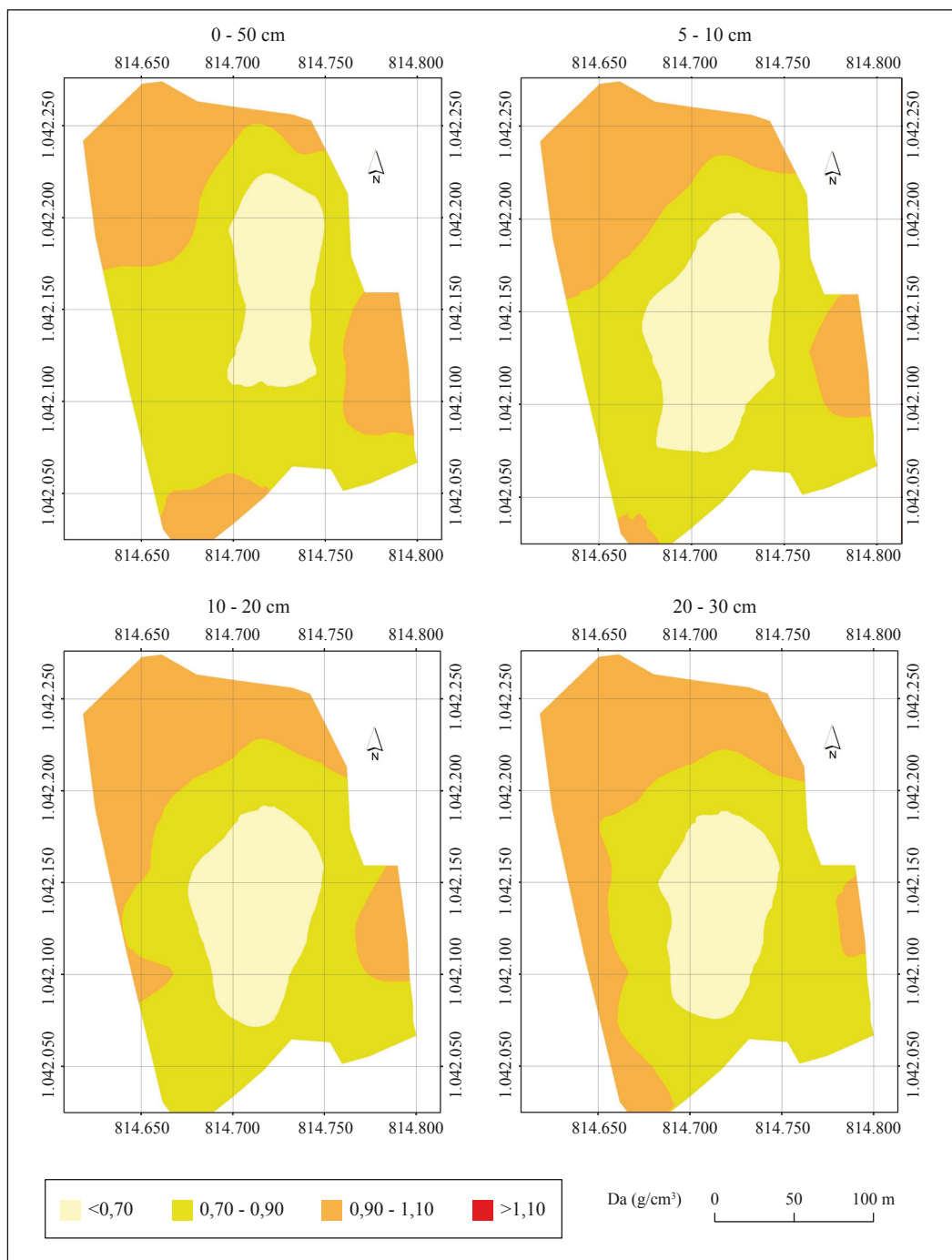
Figura 4. Mapas de variabilidad espacial de la Da para cuatro profundidades a nivel de lote cafetero ubicado en un suelo de la unidad 200.
