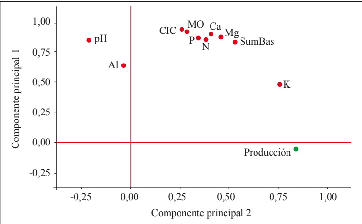
Figura 3. Análisis de Componentes Principales (ACP) de las variables químicas del suelo.
