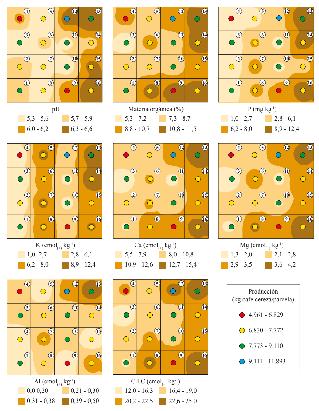
Figura 2. Distribución espacial de nutrientes en el suelo, pH y producción en un lote de 3,2 ha. Finca El Roble, municipio Los Santos, Santander-Colombia.
