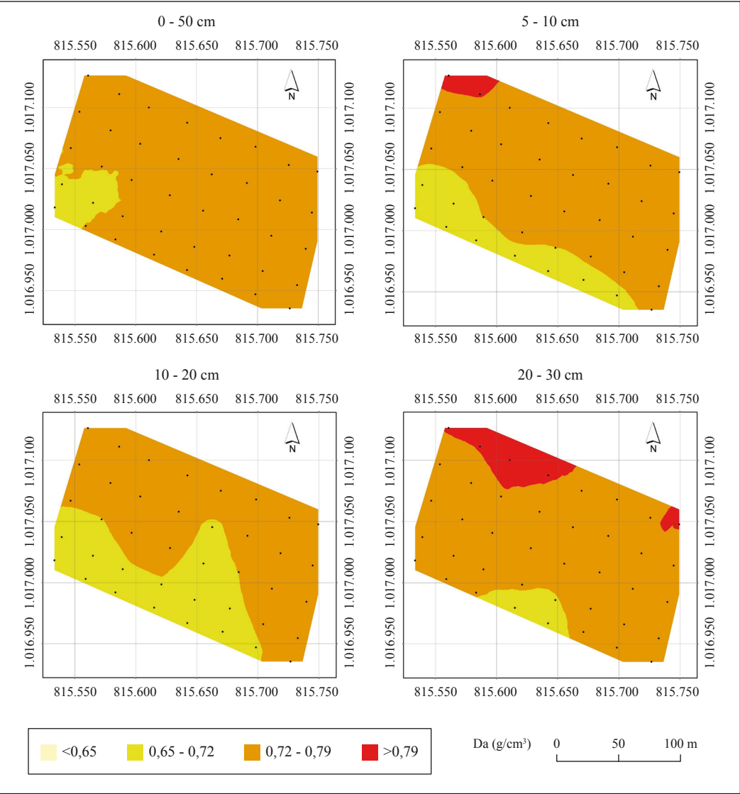
Figura 3. Mapas de variabilidad espacial de la Da para cuatro profundidades en un lote de café ubicado en suelo de la unidad Chinchiná.
