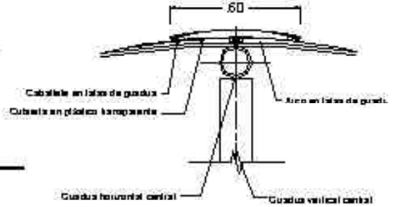
ESTRUCTURA CABALLETE DETALLE C
