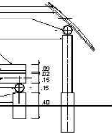
DETALLE A VISTA LATERAL CUBIERTA
