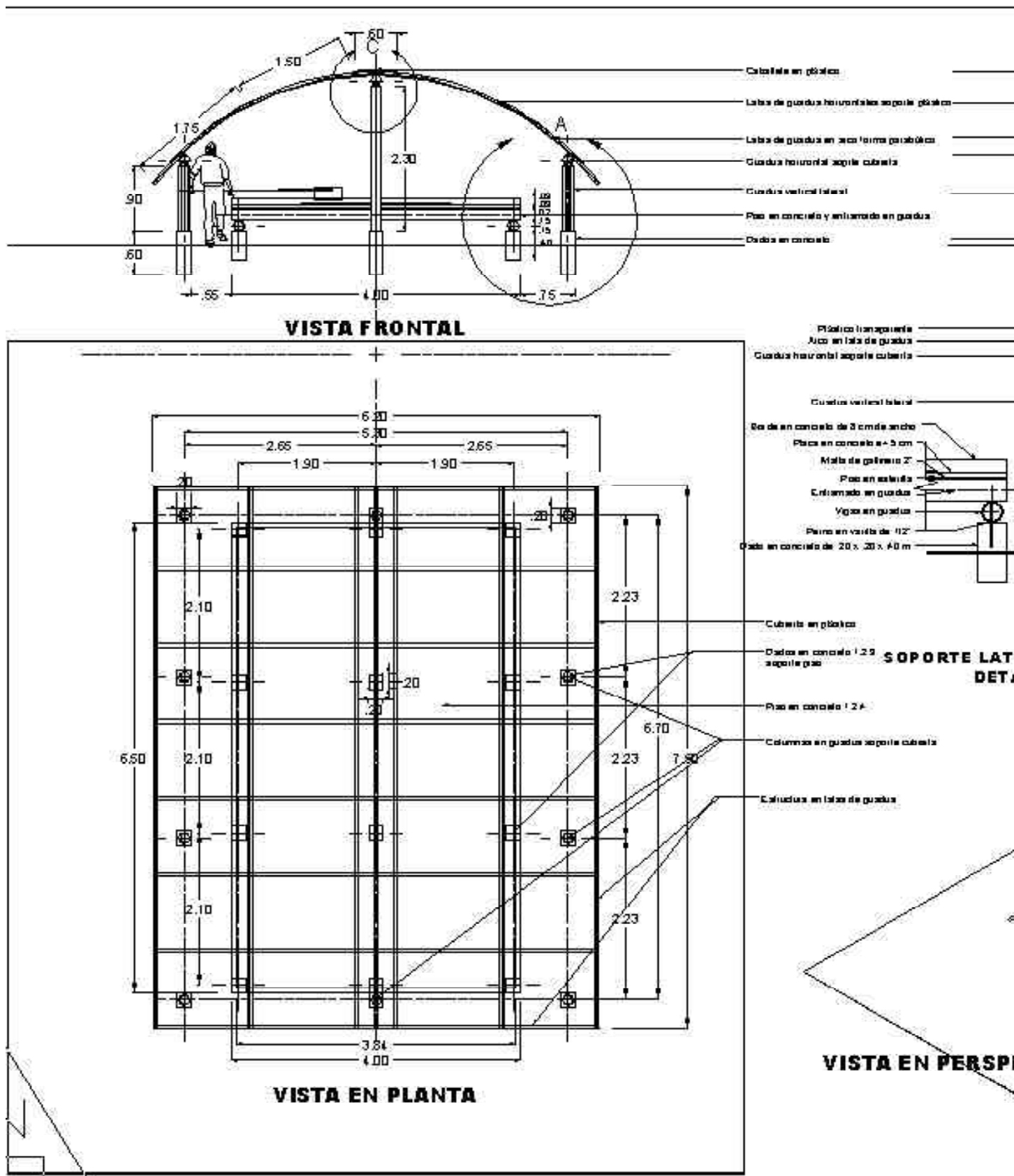
Figura3. Planos de secador solar parabólico de café
