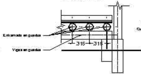
ESTRUCTURA PISO DETALLE B
