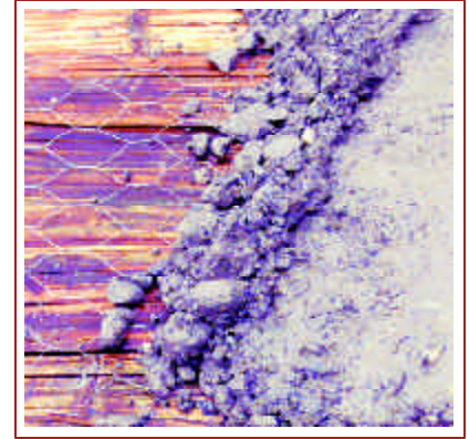
Figura 7. Concreto reforzado con malla de gallinero de 2"
